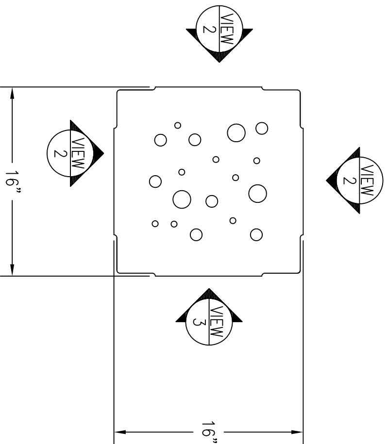
1 WS-215, STOOL TOP Scale: 1/8" = 1"
