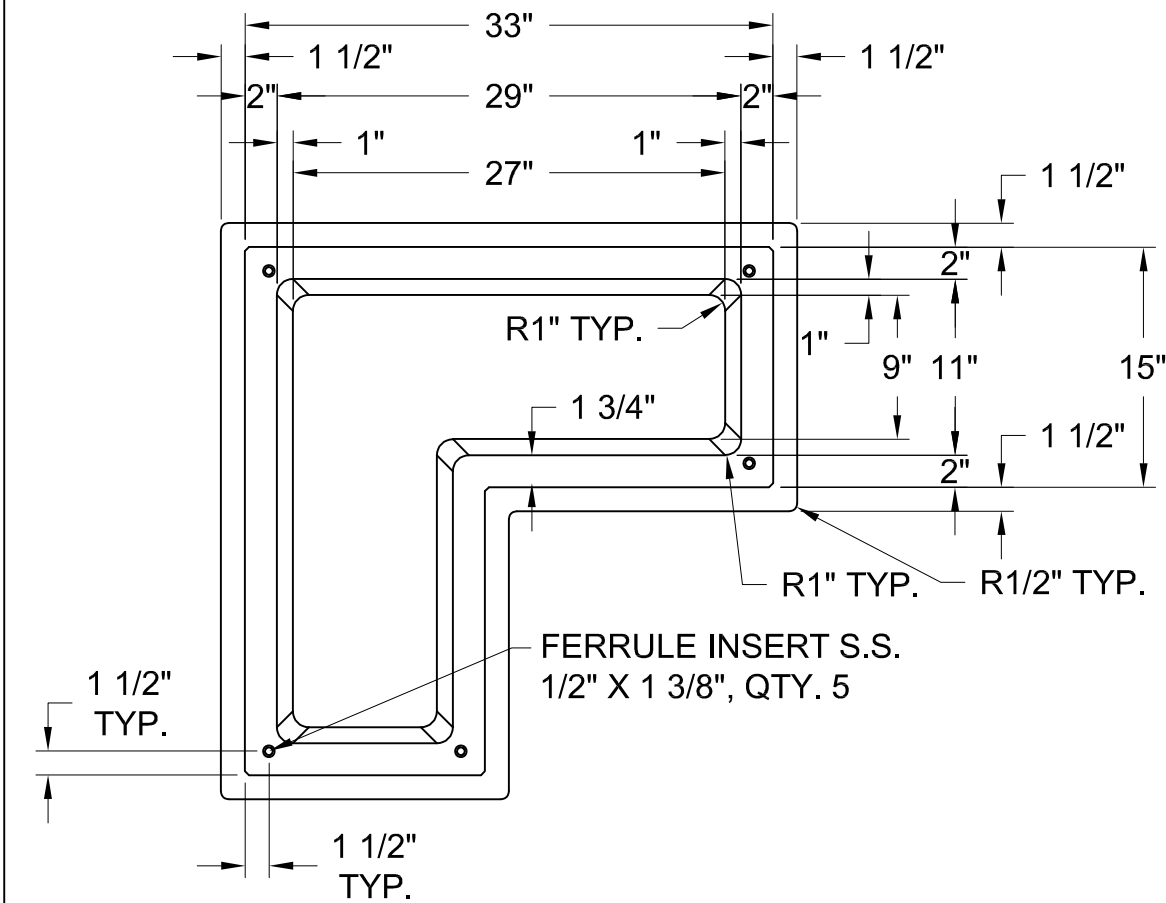
2 BOTTOM VIEW SCALE: 1" = 1'
