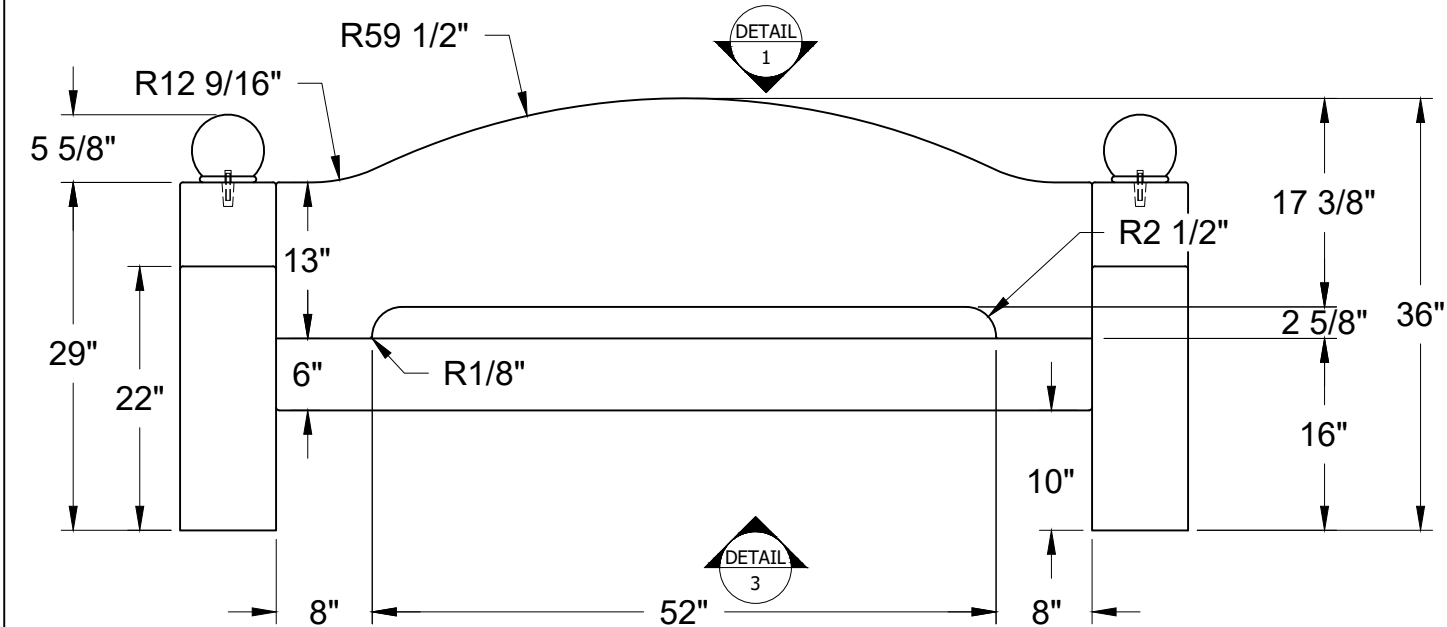
2 FRONT ELEV. SCALE: 3/4" = 1'
