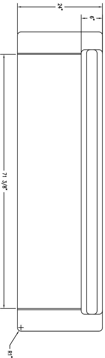
1 TOP VIEW Scale: 1/8" = 1"
