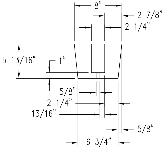
2 ELEVATION VIEW Scale: 1/8" = 1"
