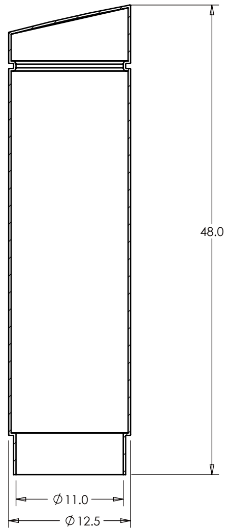
SECTION A-A
