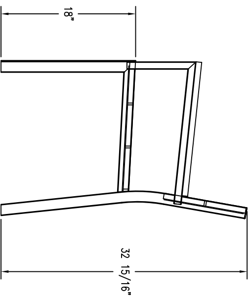
3 SECTION VIEW Scale: 1/8" = 1"
